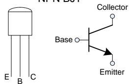
2N5088 NPN BJT
