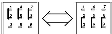
3PDT Foot Switch
